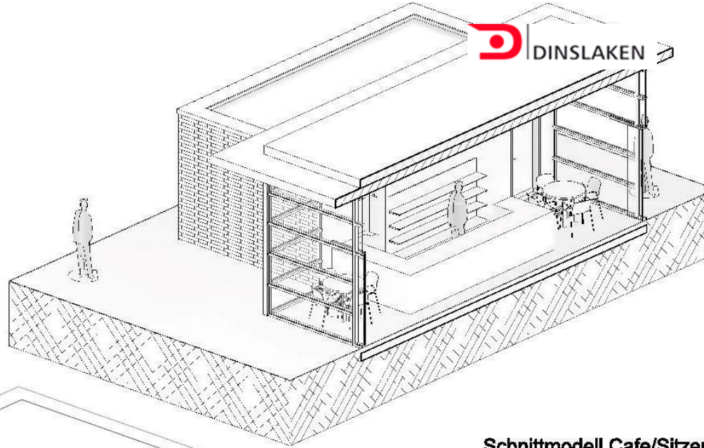
Schnittmodell Cafe/Sitzer
